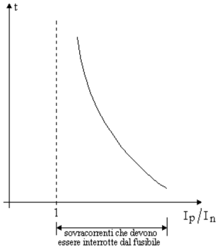
Fig.2. Esempio di caratteristica di intervento di un fusibile
