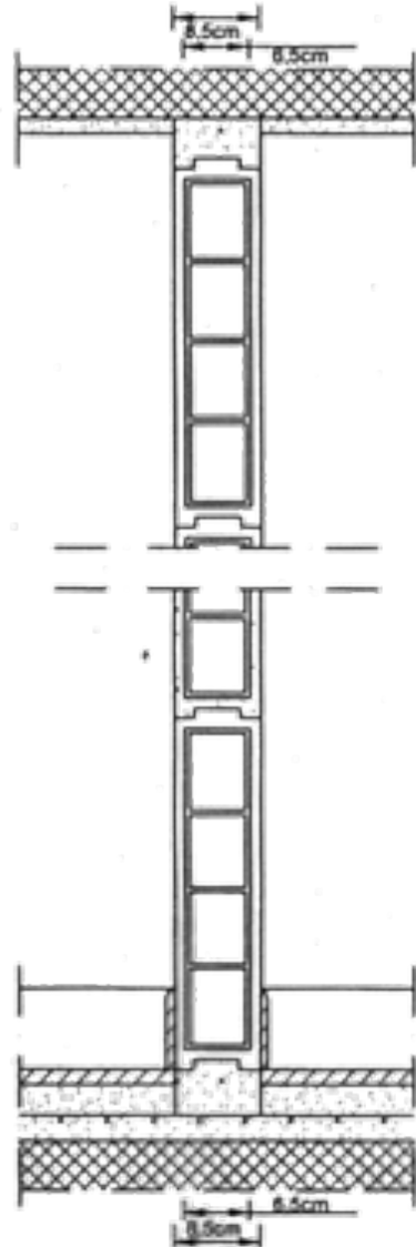
p. con blocchi in latero - gesso
