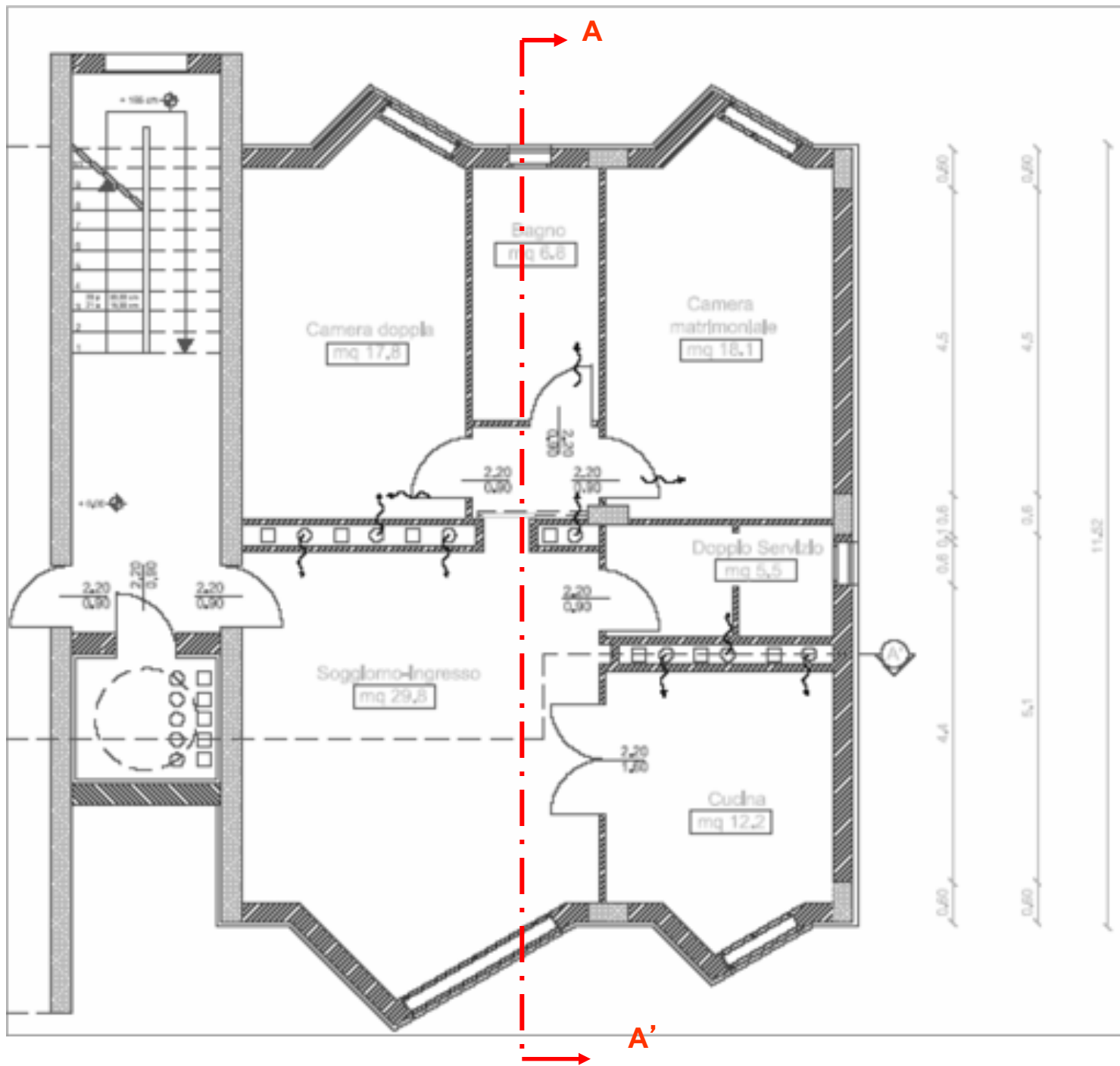
Pianta scala 1:100
