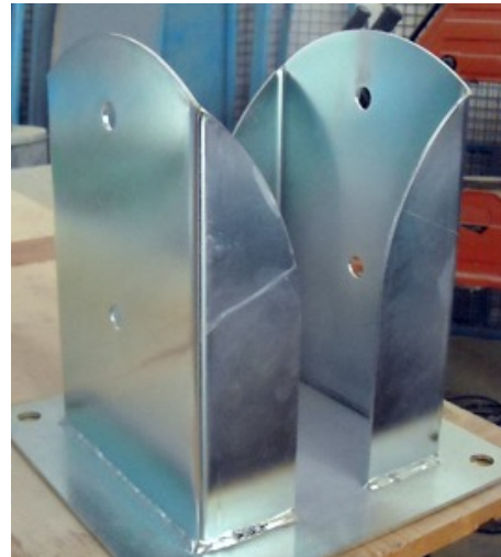
Staffa a bicchiere per pilastri
