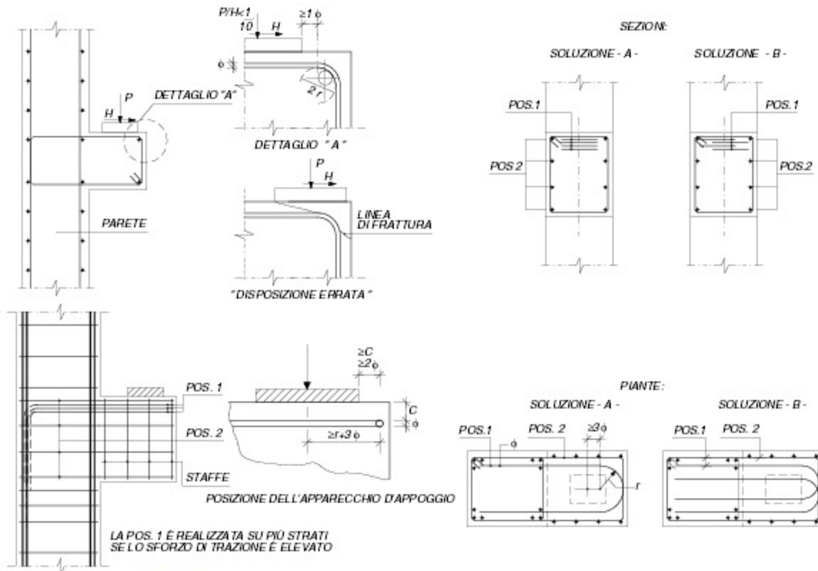
FIG. D.5.6./9 MENSOLE TOZZE - POSIZIONAMENTO E DIMENSIONAMENTO DEGLI ELEMENTI TESI E COMPRESSI
