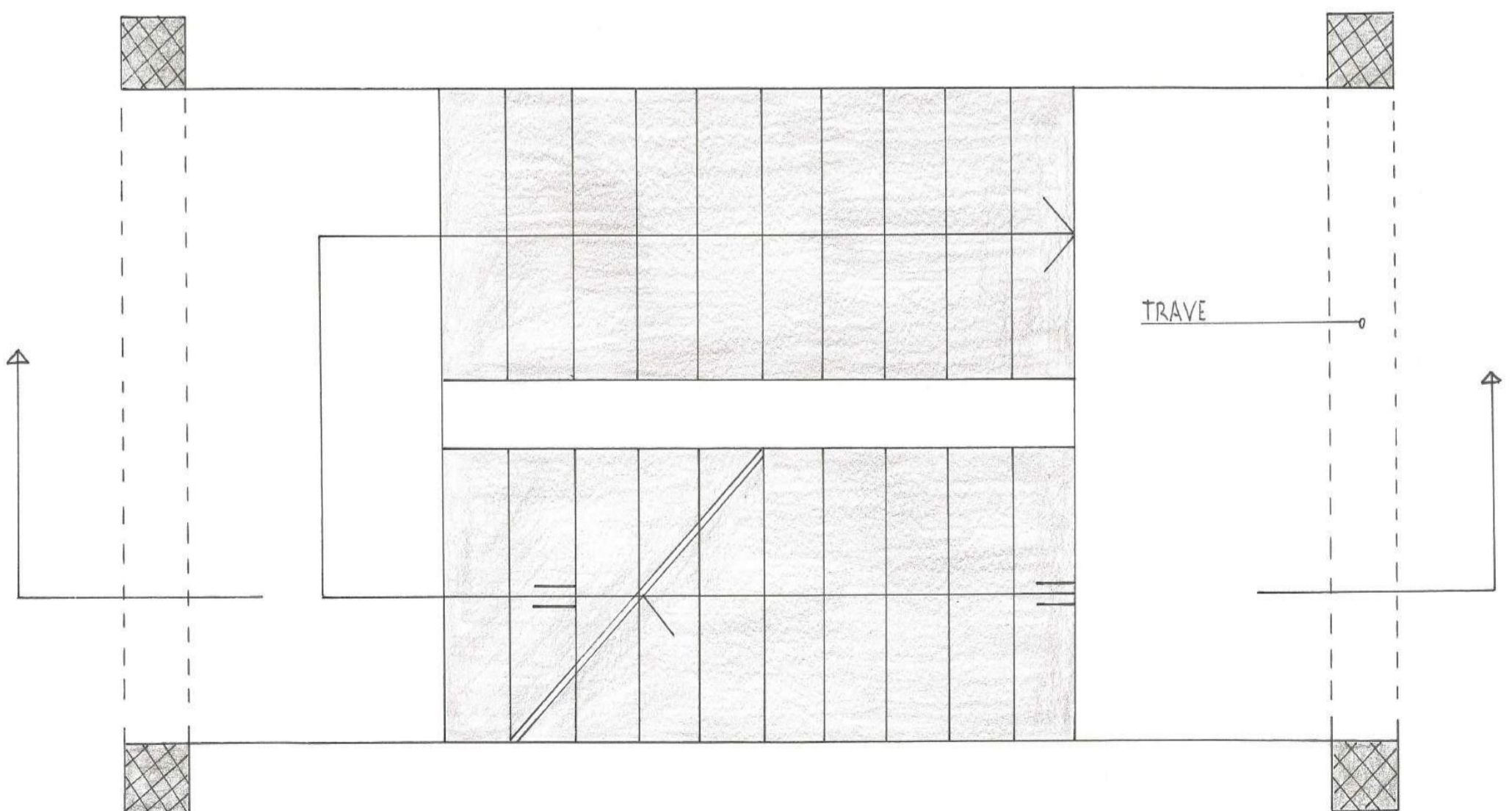
PIANTA - SCALA 1:20
